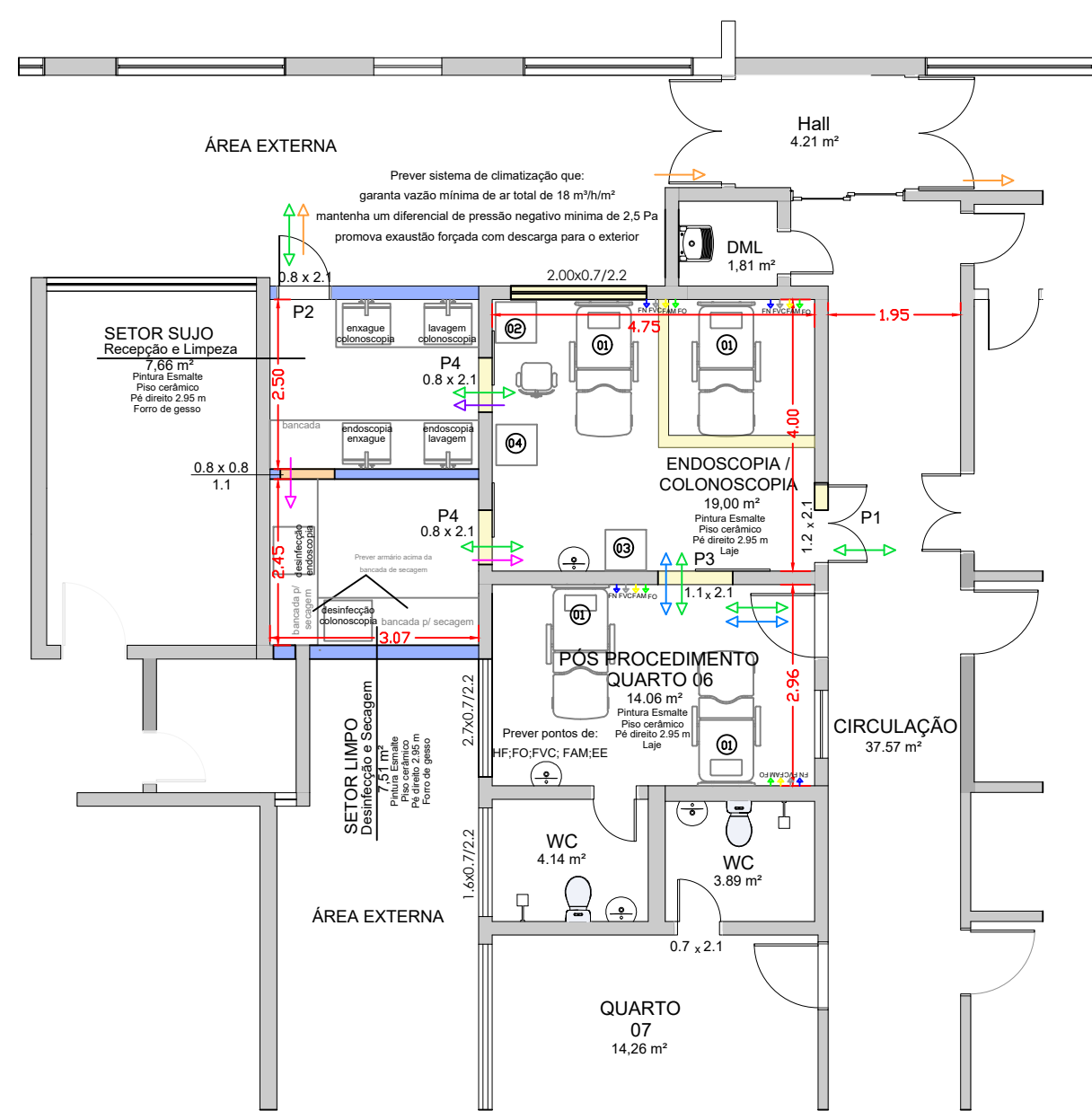
3 PLANTA DE PRETENDIDA ESCALA 1 : 100
